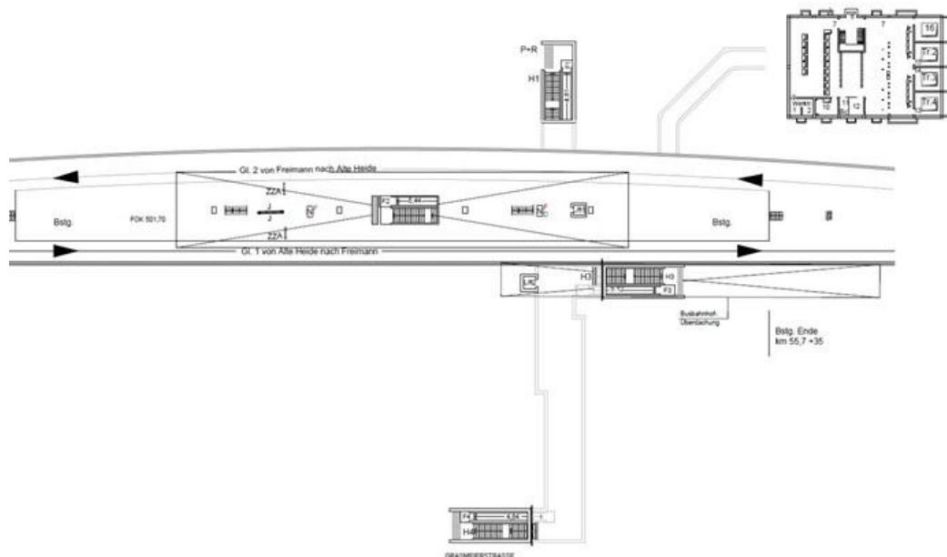
Abbildung 2: Übersicht des oberirdischen Teils des U-Bahnhofs Studententadt mit Gleichrichterwerk
