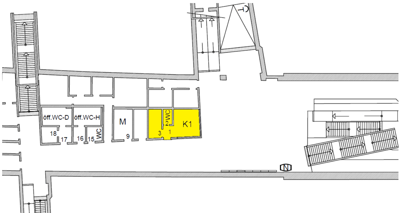
Lageplan
